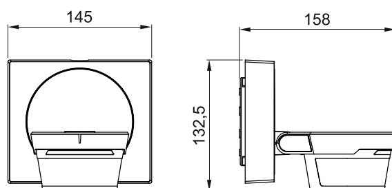
Fig. 2: Dimensions
